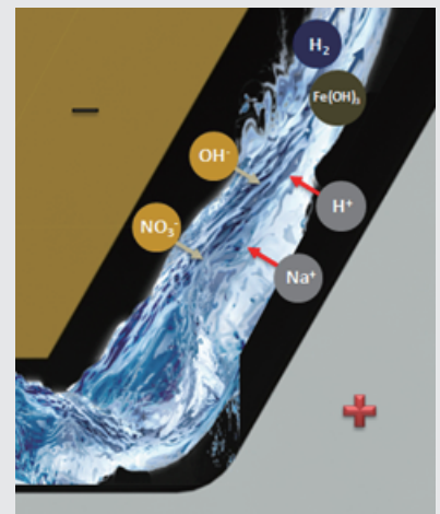
電化學加工示意圖 Electrochemical Processing Schematic
